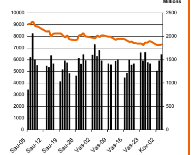
NIKKEI 225 INDEX
