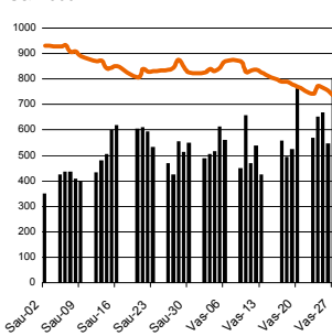
S&P 500 INDEX
