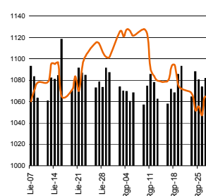
S&P 500 INDEX
