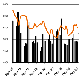
DAX INDEX
