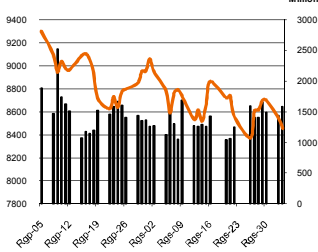
NIKKEI 225 INDEX
